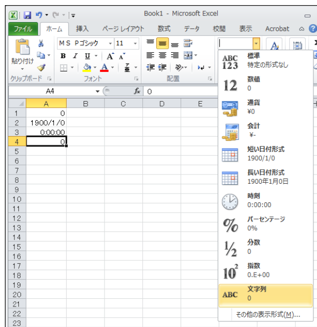
図2. 書式の変更
